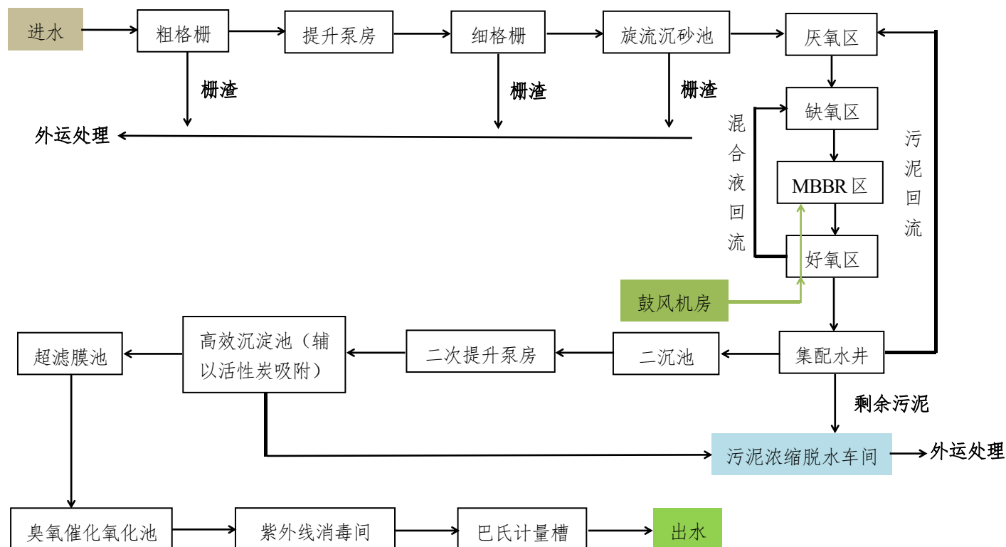
图 2.3-1 南水水质净化厂污水处理工艺流程图
